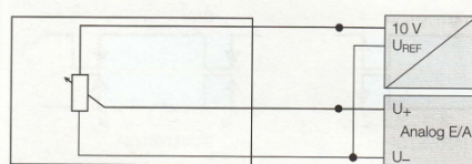
电位差计接线示意图
