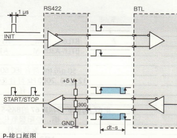
P-接口框图
