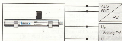
微脉冲位移传感器接线示意图
