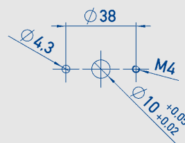
推荐孔径: 2 x \varnothing 4.3 或 2 x M4
