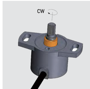
推荐孔径: 2 x \varnothing 4.3 或 2 x M4
